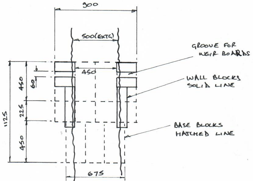
PLAN 1:20
