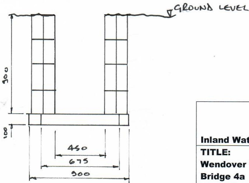
ELEVATION 1:20
